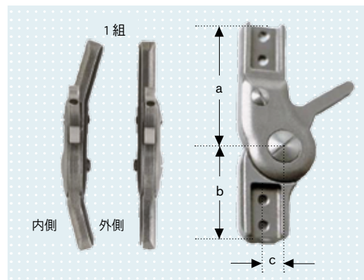
● モジュラー膝継手 ベールロック 17B23=K
